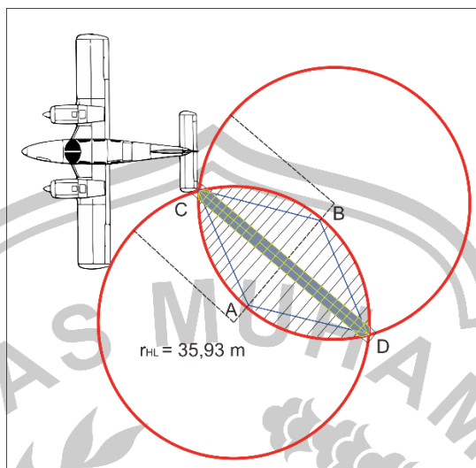
Gambar 14. Irisan Lingkaran Pada Horizontal Stabilizer Kiri
