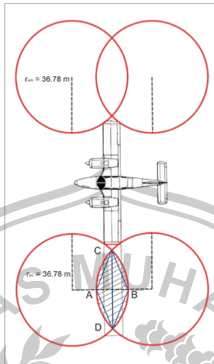
Gambar 13. Irisan Lingkaran Pada Wing Kiri dan Kanan
