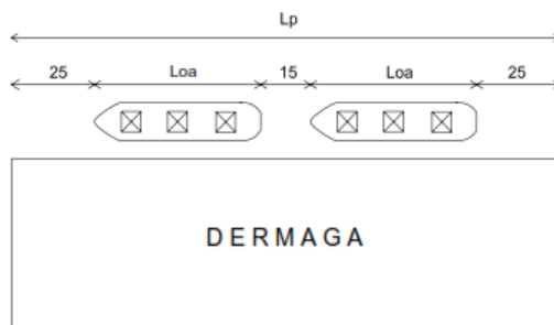
Gambar 1. Panjang Dermaga sesuai kapal yang berlabuh Sumber : Triatmodjo, 1999
