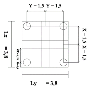
Gambar 10. struktur pondasi
