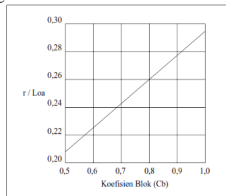
Gambar 2. Grafik koefisien blok dan Jarak sandar kapal ke pusat berat Sumber : Triatmodjo, 1999
