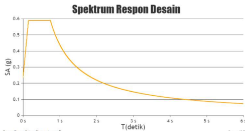
Gambar 1. Spektrum respons desain sumber : website ciptakarya
