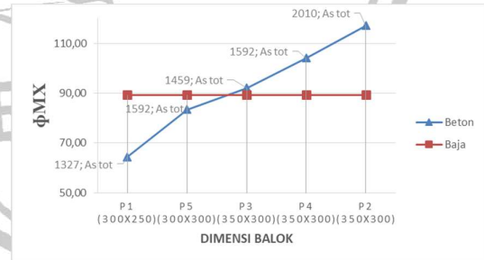
Grafik 3. Hubungan \phi M_n Beton dan \phi M_n baja sumber : perhitungan excel
