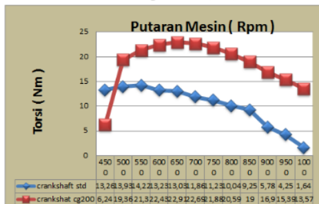
Gambar 4. Grafik Perbandingan Torsi (Nm)
