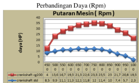
Gambar 3. Grafik Perbandingan Daya (Hp) Menggunakan Poros Engkol (Crankshaft) dan Poros Engkol (Crankshaft) CG200
