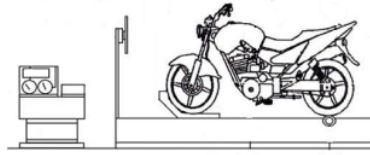
Gambar 2. Skema Alat Uji Dynotes (Dahayu, 2016:07)
