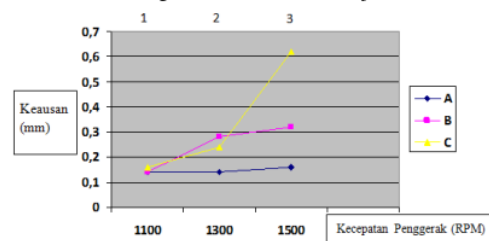
Gambar 8. Grafik Variasi Kecepatan
