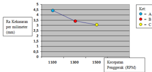
Gambar 12. Grafik Rata-Rata Tingkat Kekasaran Benda Kerja
