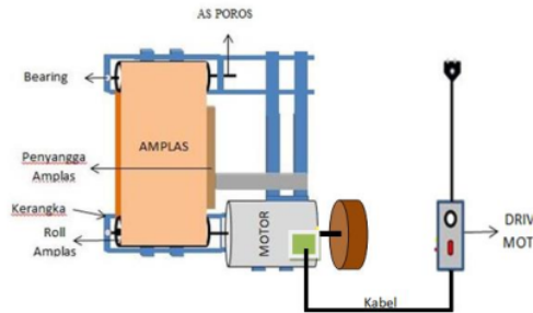
Gambar 2. Desain Perancangan Mesin
