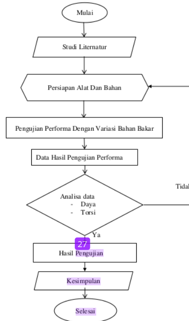
Gambar 3.1 Diagram Alir
