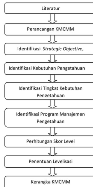
Gambar 1. Metodologi Penelitian
