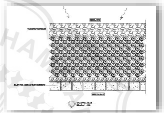
Gambar 14. Revetment tampak atas Sumber : Autocad 2021
