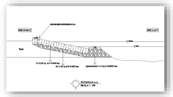
Gambar 13. Revetment potongan Sumber : Autocad 2021
