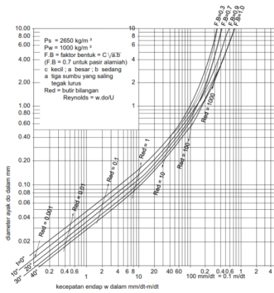
Gambar 2.7 Hubungan Antara Diameter Saringan dan Kecepatan Endap untuk Air Tenang
