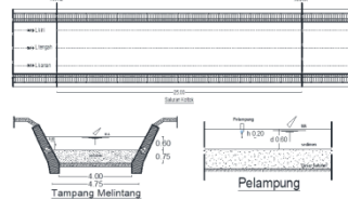
Gambar 2.10 Sketsa Alur untuk pengukuran kecepatan dan model pelampung tungkai (metode apung)
