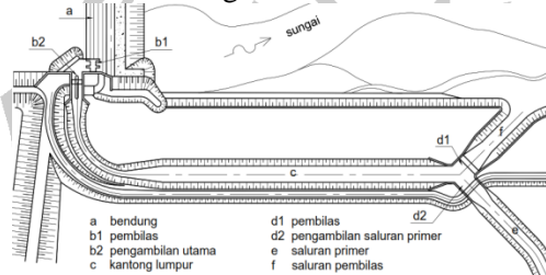
Gambar 2.1 Tipe Tata Letak Kantong Lumpur
