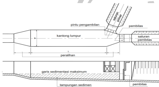
Gambar 2.2 Tata Letak Kantong Lumpur yang Dianjurkan
