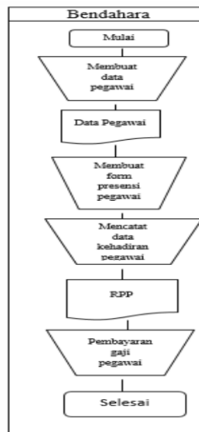
Gambar 2 Bagan Alir Flowchart
