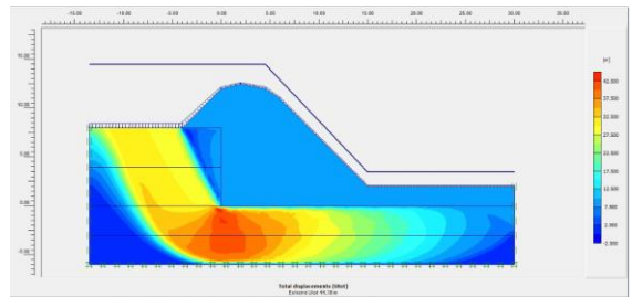
Gambar 9 garis keruntuhan bendung dengan beban luar
