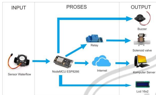
Gambar 2. Diagram Blok Sistem Sumber : Penelitian
