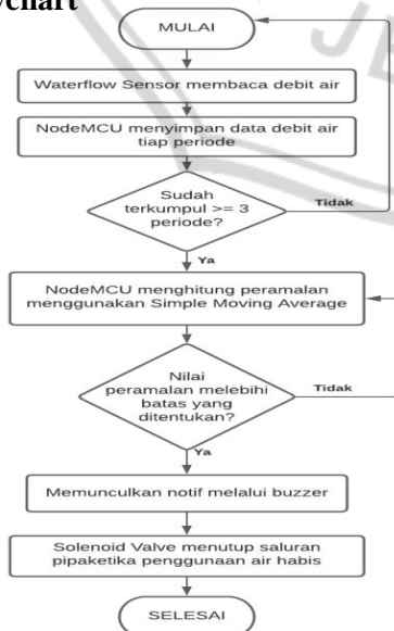
Gambar 3. Flowchart Sistem Sumber : Penelitian
