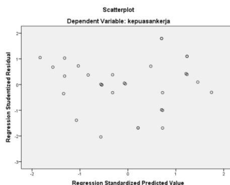
Grafik 1: Grafik Scater Plot.
