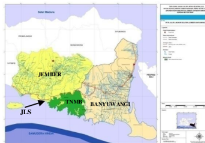
Gambar 1. Orientasi Peta Kabupaten Jember dan Banyuwangi
