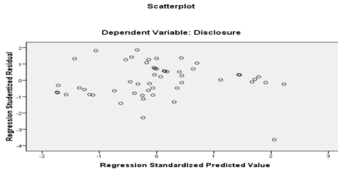
Gambar 2 Uji Heteroskedastisitas
