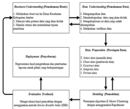
Gambar 2. Tahapan Penelitian. dengan CRISP-DM
