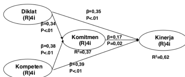
Gambar 3. Hasil Analisis Jalur
