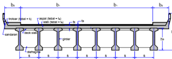
Gambar 18. Potongan Melintang Pelat Lantai Jembatan
