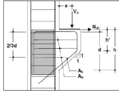
Gambar 7. Konsol Pendek
