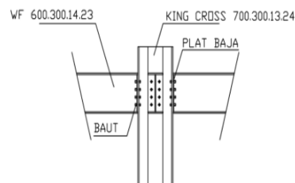
Gambar 3.4 Sambungan Kolom – Balok tampak Depan Samping
