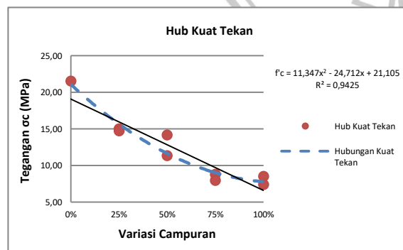
Gambar 2. Hubungan Kuat Tekan dengan Variasi Campuran BAS 0%, 25%, 50%, 75% dan 100%.
