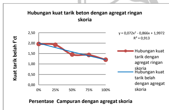
Gambar 4. Hubungan Kuat Tarik Belah Beton Dengan Agregat Skoria.
