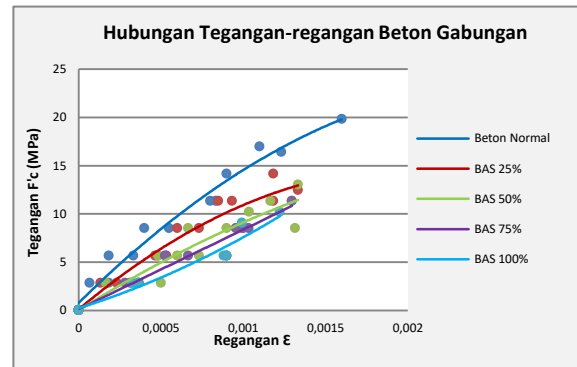
Gambar 3. Hubungan Tegangan - Regangan Beton Gabungan.
