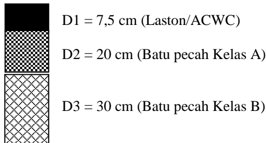
Gambar 7. Tebal Lapisan Perkerasan (hasil perhitungan)
