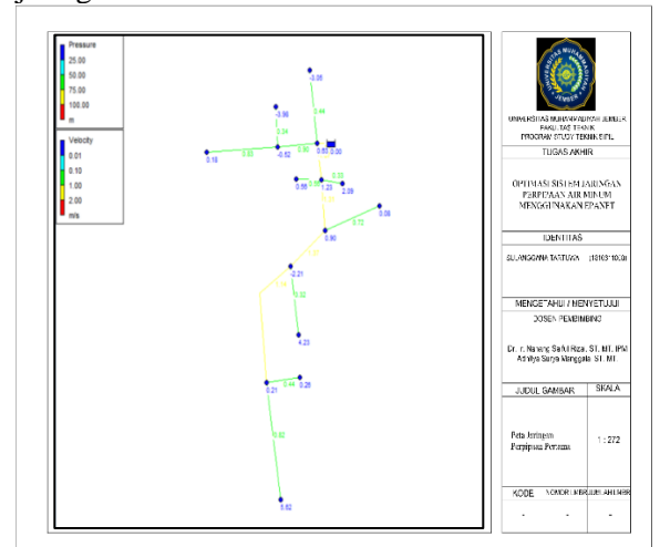
Gambar 7 Peta Jaringan Perpipaan Pertama Bila Tanpa Menara Air Sumber: Software Epanet 2.2, 2022 Peta jaringan pertama pada node 15, 14 dan
