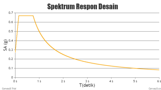
Gambar 5. Spektrum respons desain (Sumber : http://rsa.ciptakarya.pu.go.id/2021 )
