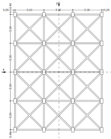
Gambar 13. Gambar strip dalam arah x dan y (Sumber: Gambar autocad 2012)
