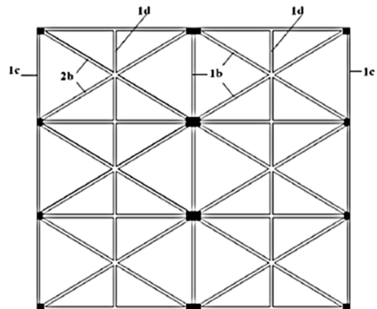
Gambar 2. Tampak Atas Pondasi KSSL (Sumber : Kinanthi, 2016)
