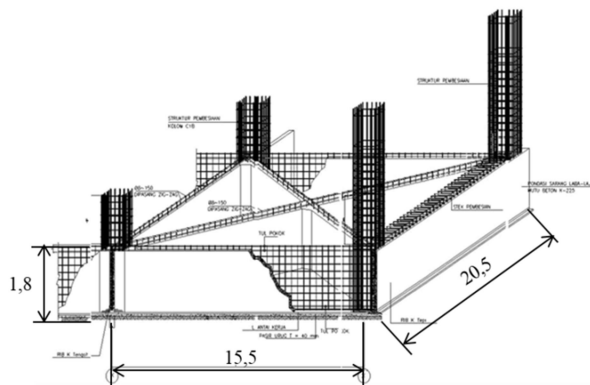
Gambar 10. Isometrik Pondasi KSSL (Sumber: Dokumentasi PT. Katama Suryabumi, 2008)
