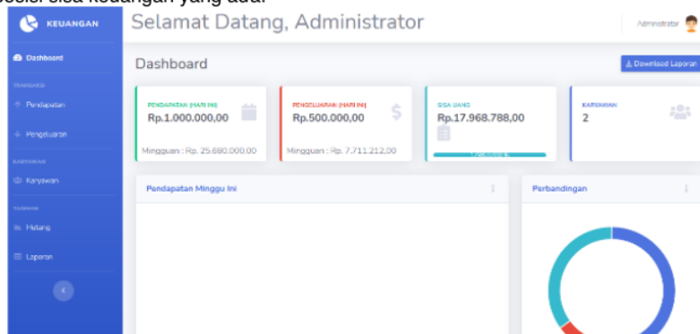
Gambar 8 Halaman Utama
