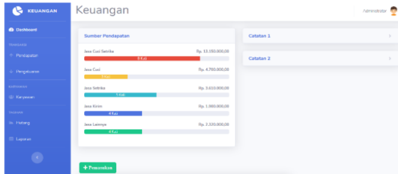
Gambar 9 Halaman Rekapitulasi
