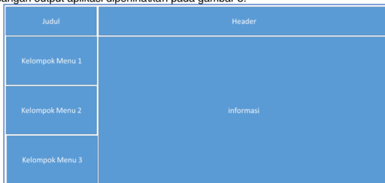
Gambar 5. Perancangan Antarmuka
