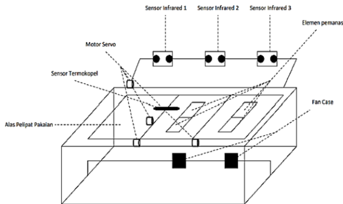
Gambar 6. Desain Mekanik Alat
