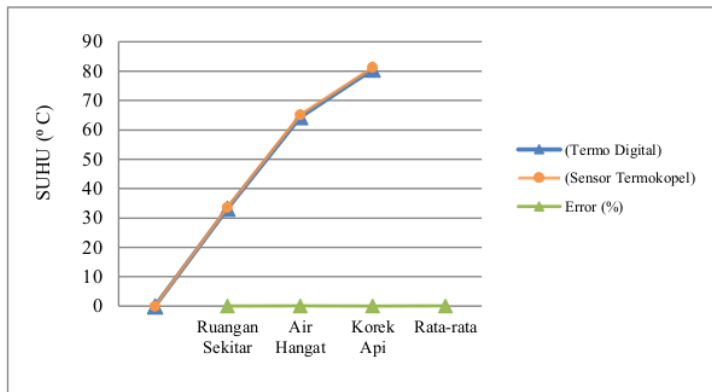
Gambar 10. Grafik Pengujian Sensor Termokopel
