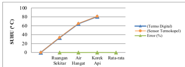
Gambar 8. Grafik Pengujian Sensor Termokopel
