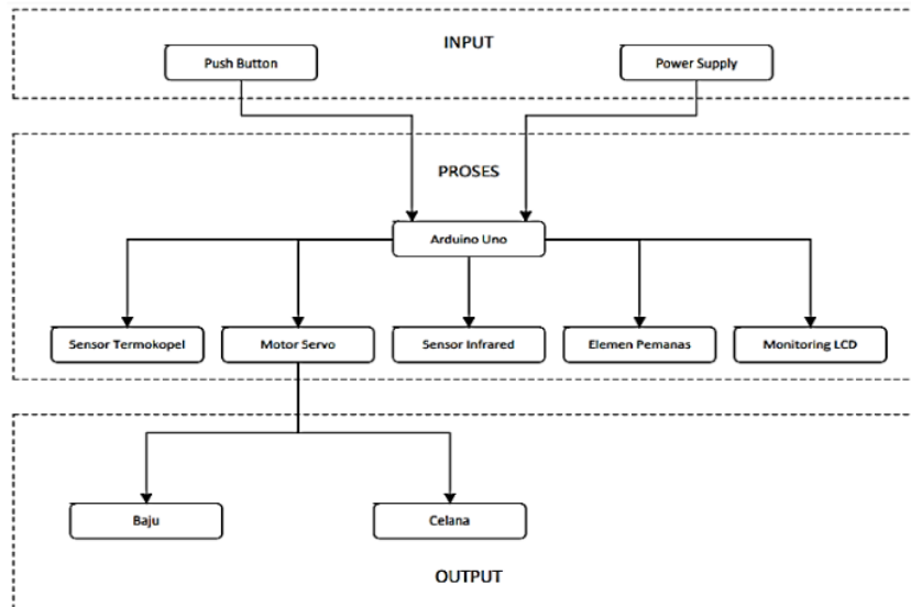
Gambar 4. Blok Diagram Sistem
