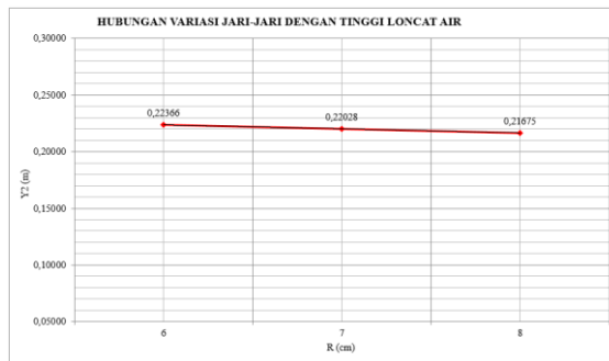
Gambar 17. Hubungan Antara Variasi Jari - jari (cm) dengan Tinggi Loncatan Air (m) hasil uji lapangan
