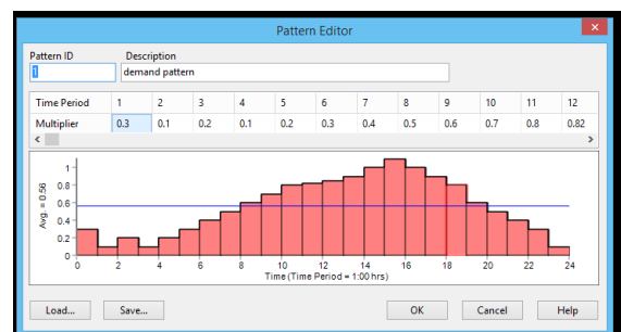
Gambar 11. grafik jam puncak dan kebutuhan air setiap jam selama 24 jam dari jam 00.00 – 12.00 model 1
