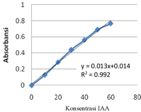
Gambar 2. Kurva standar IAA
