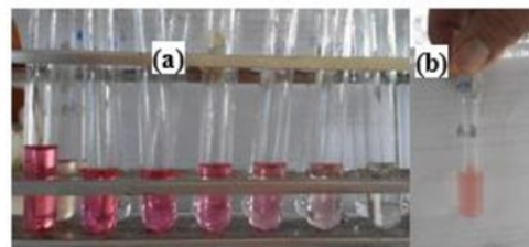
Gambar 1. Pengukuran konsentrasi IAA secara kualitatif menggunakan metode kolorimetri. Ket. (a) Konsentrasi standar IAA sintetik (0-60 ppm), (b) Sampel kultur Bacillus sp.
