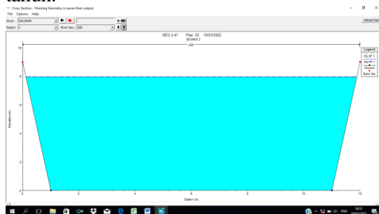
Gambar 8 Ketinggian Muka Air Dimensi Eksisting Trapezium
