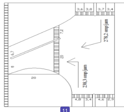
Gambar 5.5. volume arus lalu lintas pada saat kereta api melintas (real)
