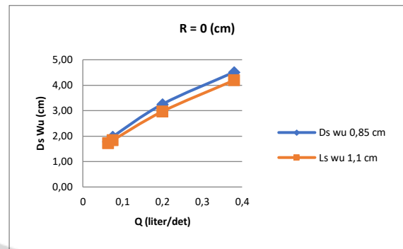
Gambar 16. Grafik Pendangkalan Wu 0
