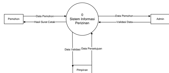
3.2 Diagram Konteks
