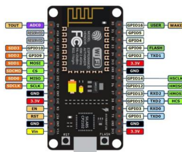
Gambar 2. NodeMCU esp2866 beserta pinnya
