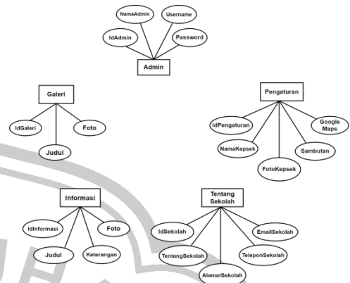
Gambar 7. ERD website profil sekolah SD Negeri Kalidilem 03. Sumber: Penulis, 2024.
