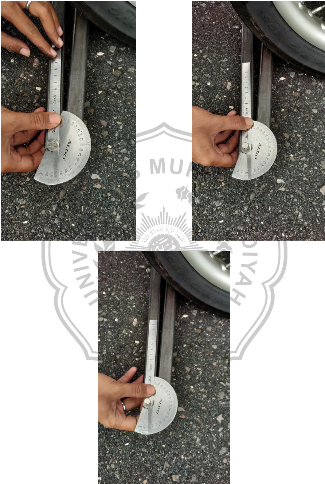
Lampiran 5. Pengukuran sudut kemiringan dengan tekanan ban 25 Psi
