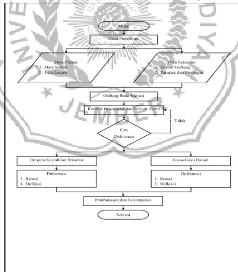
Gambar 3.4 Kerangka Penelitian
