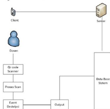
Gambar 11 Arsitektur Sistem pada Platform Android
