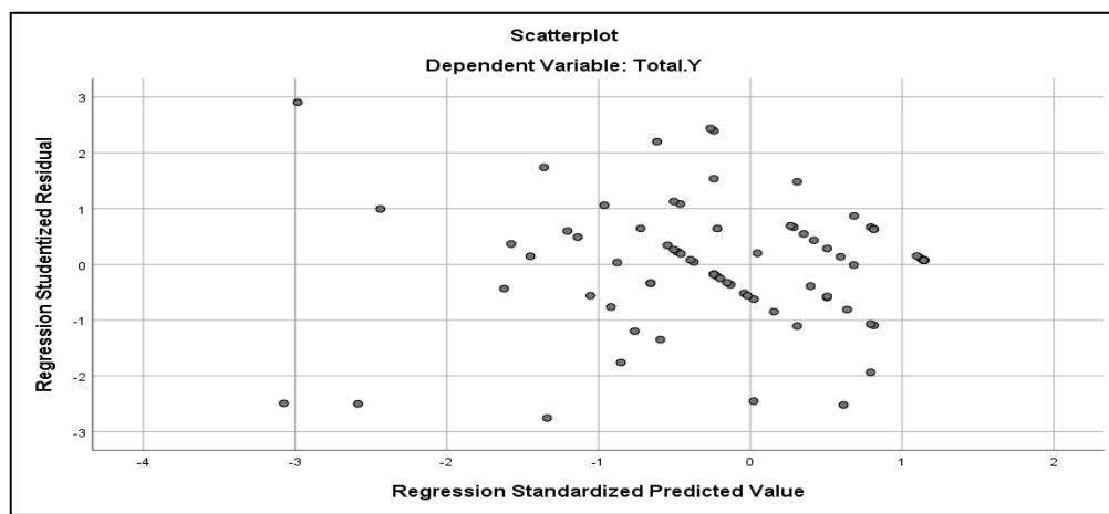
Gambar 2. Uji Heteroskedastisitas
