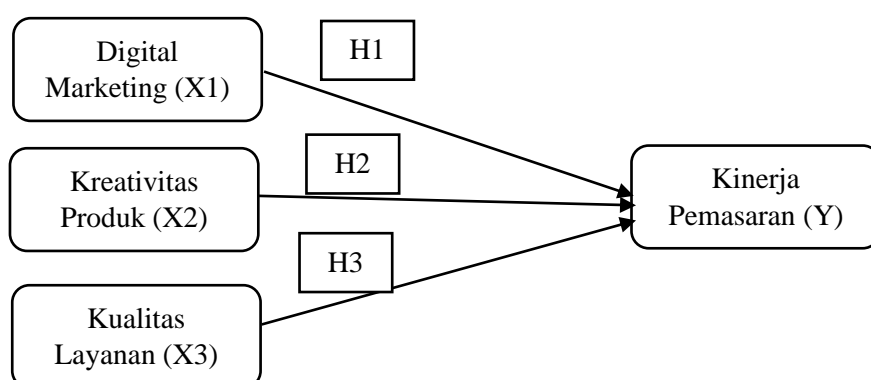
Gambar 2. Kerangka Pemikiran
