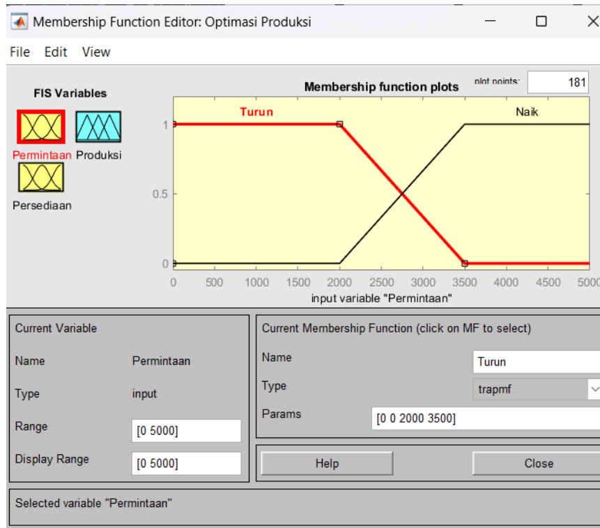
Gambar 6. Himpunan Fuzzy Variabel Permintaan
