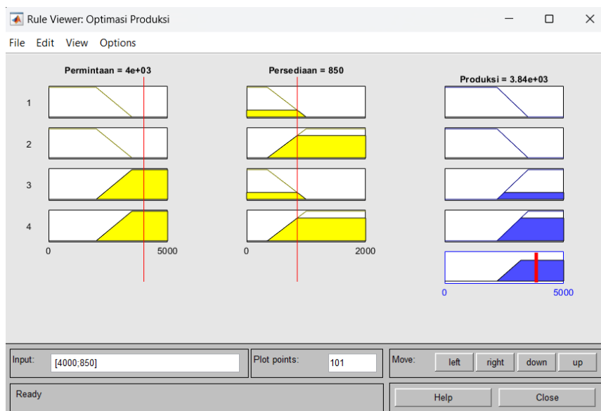
Gambar 10. Hasil Defuzzifikasi Pada Fuzzy Inference System
