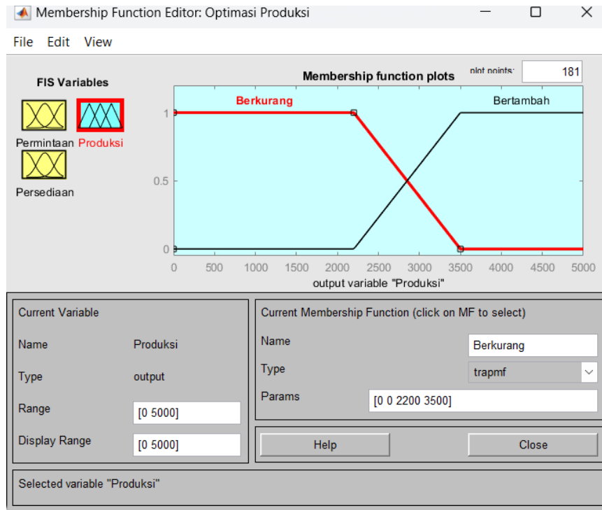
Gambar 8. Himpunan Fuzzy Variabel Produksi
