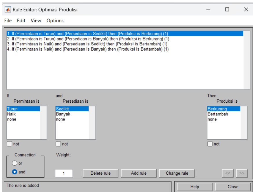
Gambar 9. Komposisi Aturan Implikasi Fuzzy yang Berlaku
