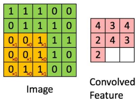
Gambar 1. Operasi Konvolusi
