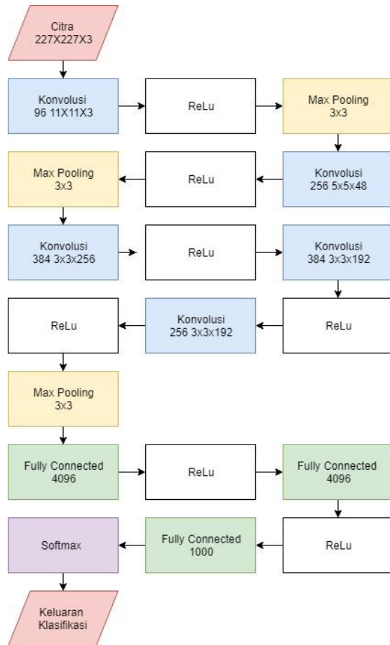
Gambar 4. Arsitektur Alexnet
