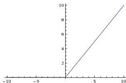
Gambar 3. Aktivasi ReLU
