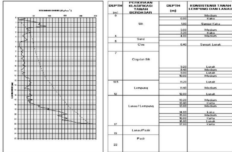
Gambar 6. Grafik Sondir dan Konsistensi tanah Sondir 2
