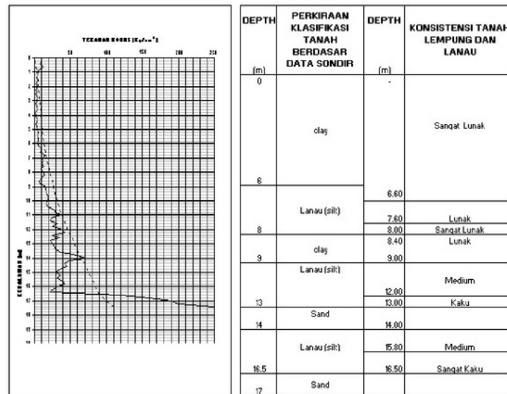
Gambar 5 Grafik Sondir dan Konsistensi tanah Sondir 1
