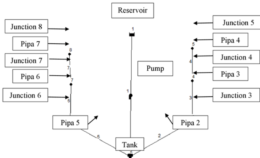
Gambar 4.2 Jaringan Distribusi Air Bersih
