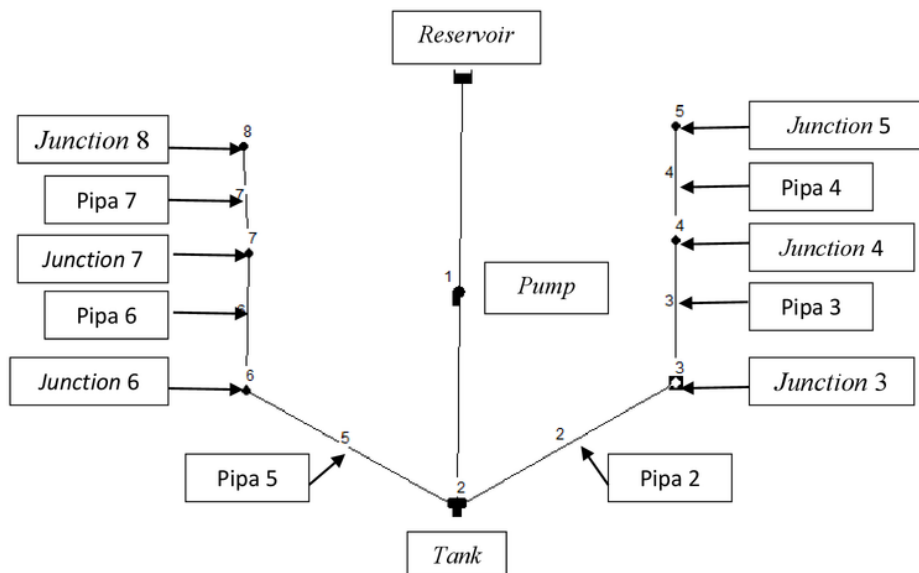
Gambar 2.1 Gambar Jaringan Distribusi Air Bersih Dalam Epanet Versi 2.0
