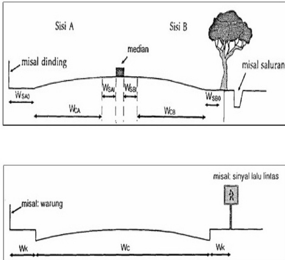
Gambar 2.1 Sketsa Melintang jalan
