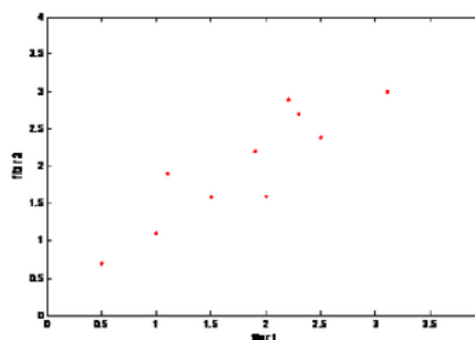
Gambar 1. Plot Grafik untuk data
