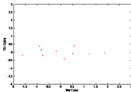
Gambar 2. Plot Grafik untuk data setelah di-PCA
