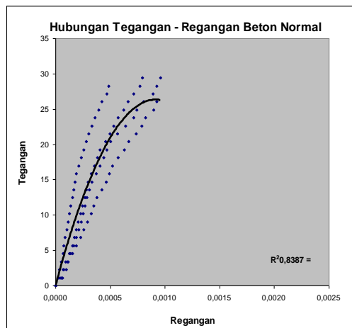
Gambar 1. Hubungan Tegangan - Regangan Beton Normal
