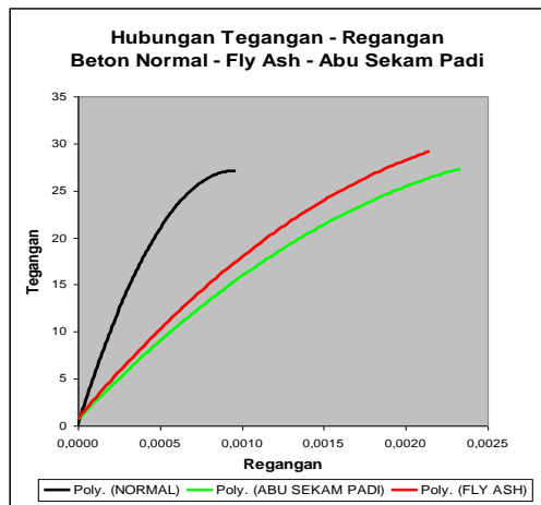
Gambar 4. Hubungan Tegangan - Regangan Beton Normal - Fly Ash - ASP
