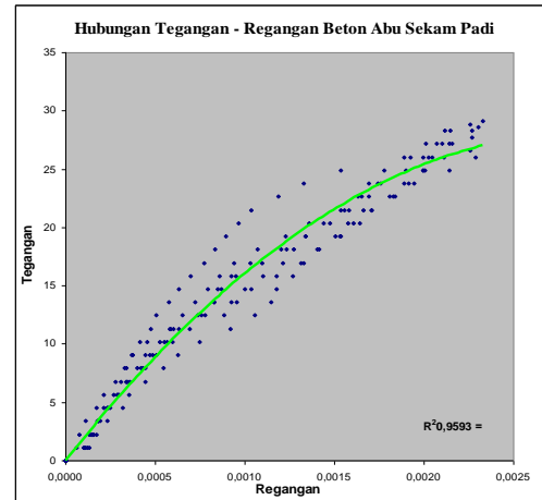
Gambar 3. Hubungan Tegangan - Regangan Beton ASP
