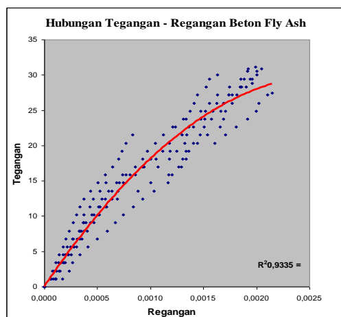
Gambar 2. Hubungan Tegangan - Regangan Beton Fly ash
