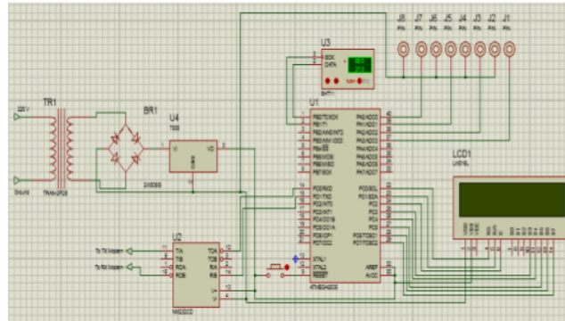
Gambar 2. Rangkaian Keseluruhan
