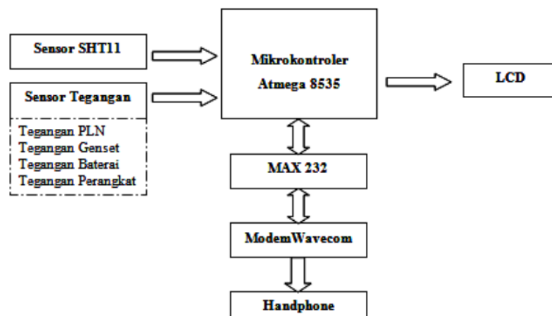
Gambar 1. Diagram Blok Sistem Kerja Alat
