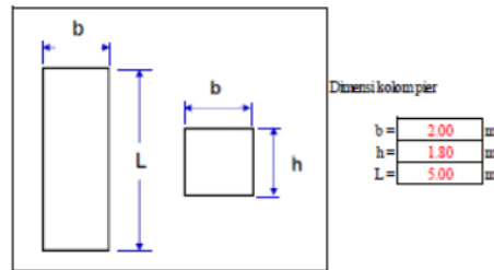
Gambar 8. Dimensi Kolom Pier Sta. 0+400
