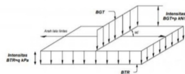
Gambar 3. Beban Lanjur D, Konfigurasi BGT dan BTR (SNI 1725 Tahun 2016)
