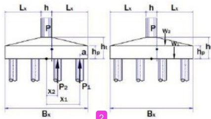
Gambar 9. Pile Cap Arah-x
