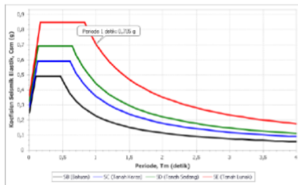
Gambar 2.9. Kurva Respon Spektrum Tanah Lunak pada Lokasi Fly over Sta 0+000 – 2+971
