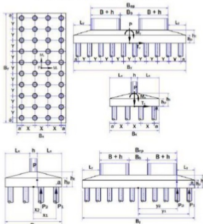
Gambar 10. Pile Cap Arah-y
