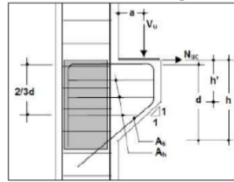
Gambar 7. Konsol Pendek
