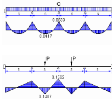
Gambar 17. Konfigurasi Pembebanan dengan Tumpuan Monolit ( s = 6 meter)
