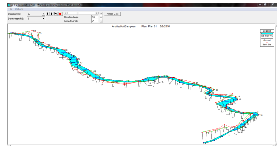
Gambar 5. Tampilan 3D Situasi Sungai Sampean Dengan Kalan Ulang 5 Tahun.
