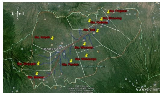
Gambar 2. Polygon Thiessen DAS Sampean Menggunakan Aplikasi Google Earth
