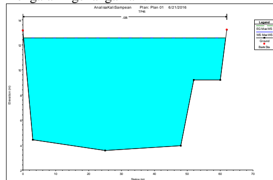
Gambar 7. Profil Melintang Penampang River Sta. 45 (Normalisasi)
