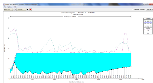
Gambar 8. Profil Muka Air Sungai Sampean ( Normalisasi )
