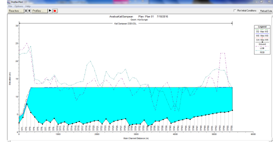
Gambar 4. Profil Muka Air Sungai Sampean (Eksisting).
