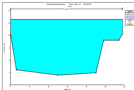
Gambar 6. Profil Melintang Penampang River Sta. 45 (Eksisting)
