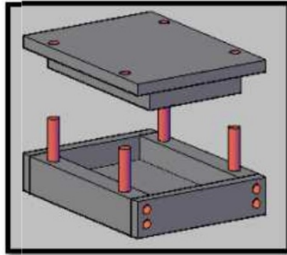
Gambar 4. Cetakan Tekan ( Compression Molding )
